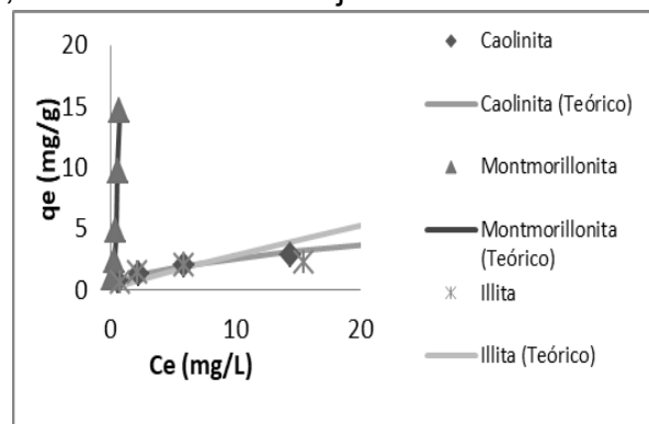
Figura 1: Cantidad de Cd(II) adsorbido por unidad de masa ( q_e ) en función de la concentración de equilibrio, C_e (mg/L) a 22°C.
