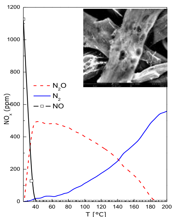
Desempeño catalítico y micrografías SEM de las fibras CMFE.Pd preparadas.
