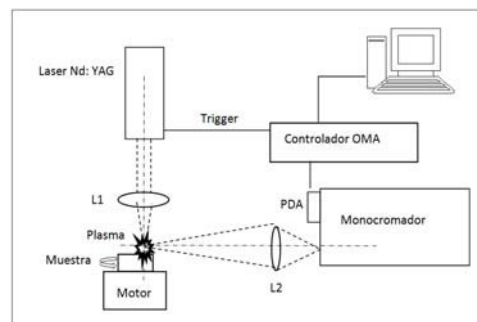
Arreglo experimental LIBS
