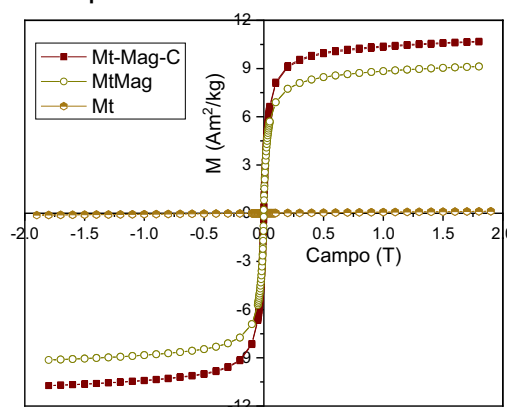
Figura: Ciclos de histéresis de las muestras indicadas.
