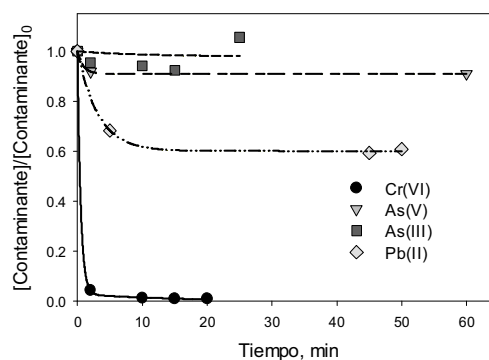
Remoción de contaminantes con NPs verdes. RM Cr(VI):Fe 1:3; As(V):Fe 1:30; As(III):Fe 1:30; Pb(II):Fe 1:30.
