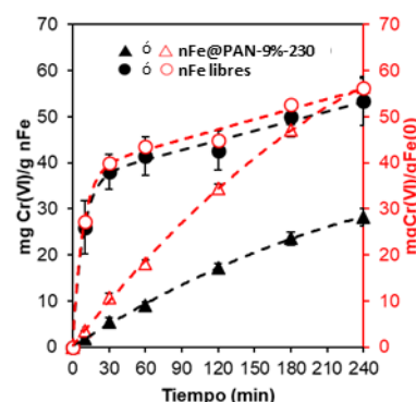
Fig 1. Eficiencia de eliminación de Cr(VI) por gramo de nFe y Fe (0) en función del tiempo para nFe libres y nFe@PAN-9% -230
