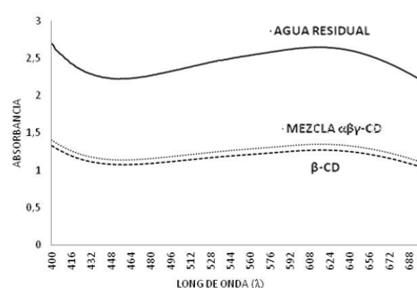
Espectro de absorción de agua residual y agua residual tratada con \beta -CD y una mezcla de \alpha\beta\gamma -CD
