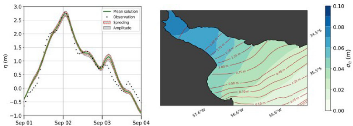
Pronóstico provisto por el sistema preoperativo para un evento de sudestada en 2010. El campo es para el pico máximo de la tormenta, donde las isolíneas indican el nivel del mar y los contornos su incerteza.
