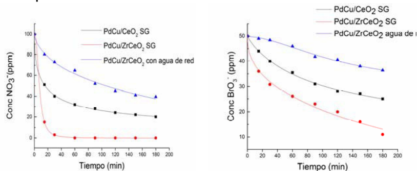
Eliminación de \text{NO}_3^- y \text{BrO}_3^- en agua destilada y agua de red
