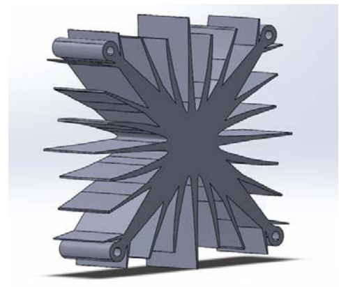
Figura 1. Pieza diseñada por optimización topológica.
