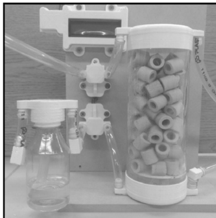
Figura 1. Estación de trabajo operacional, para la práctica de absorción de etanol en agua.
