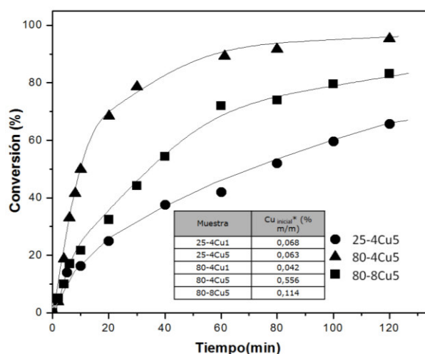
Figura 1. Conversión de Fenol en función del tiempo.
