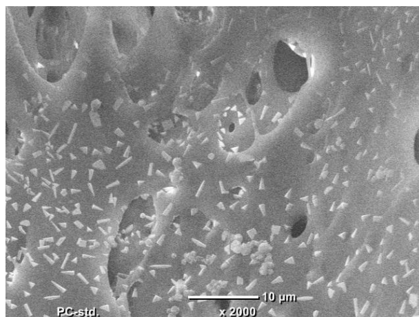
Micrografía electrónica de halloysitas tubulares
