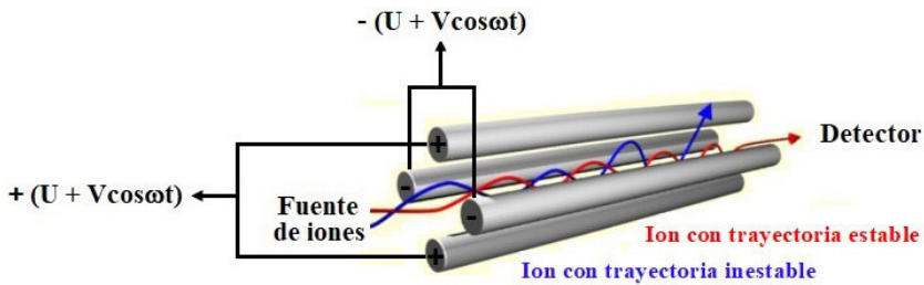
Figura N.º 8. Funcionamiento de un cuadrupolo.
