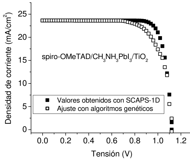
Figura 7. Característica corriente-tensión para la validación del modelo.
